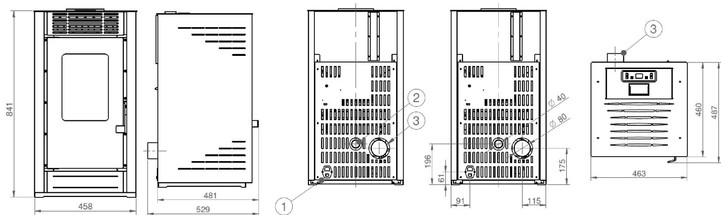
LEGENDA: 1- Interruptor e tomada de alimentação | 2- Entrada de ar | 3- Saída fumos
